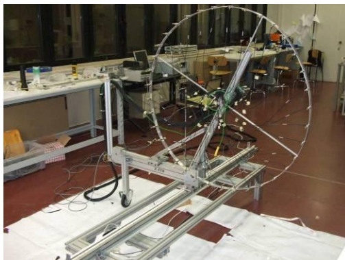
36 microphones array
