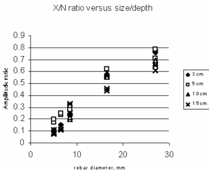
Abbildung 4.1.3: Quotient der beiden Reflexionsstärken in Abhängigkeit vom Durchmesser und der Tiefe (aus Utsi, 2004)
