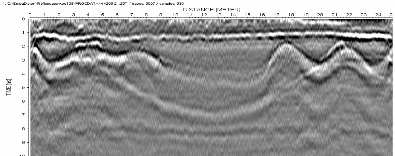
Abbildung 5.3.4: Datensatz von der Überführung Wyssenried
