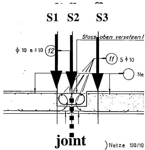
Abbildung 5.3.7: Überführung Burggasse, Schnittpositionen im Detail
