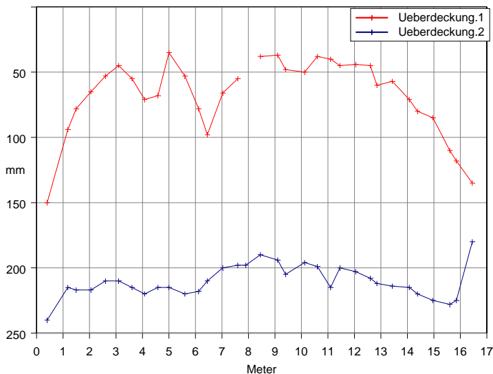
Abbildung 10.5.9: Eisenüberdeckung der beiden Bewehrungslagen entlang der Linie A
