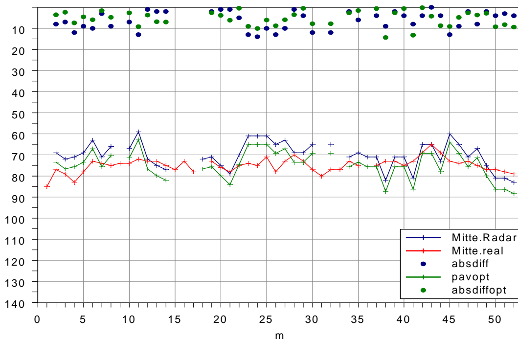
Abbildung 10.1.18: Radarergebnis und Realität für die Asphaltstärke auf der Spur Mitte, S2
