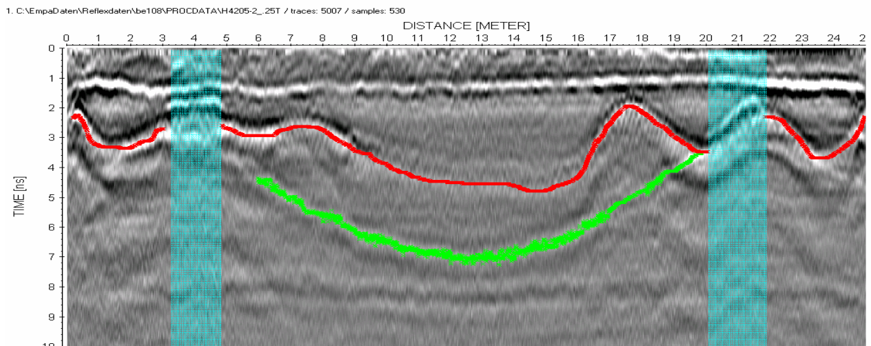
Abbildung 5.3.5: Datensatz von der Überführung Wyssenried mit eingezeichneten Reflexionen, rot=oberste Bewehrungslage, grün=benachbartes Vorspannkabel, blau=Bereiche in denen keine Eisenüberdeckung bestimmt werden konnte
