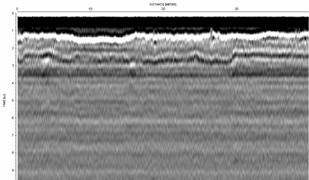
Abbildung 10.2.8: Radardaten der Linie B, Antennen quer montiert
