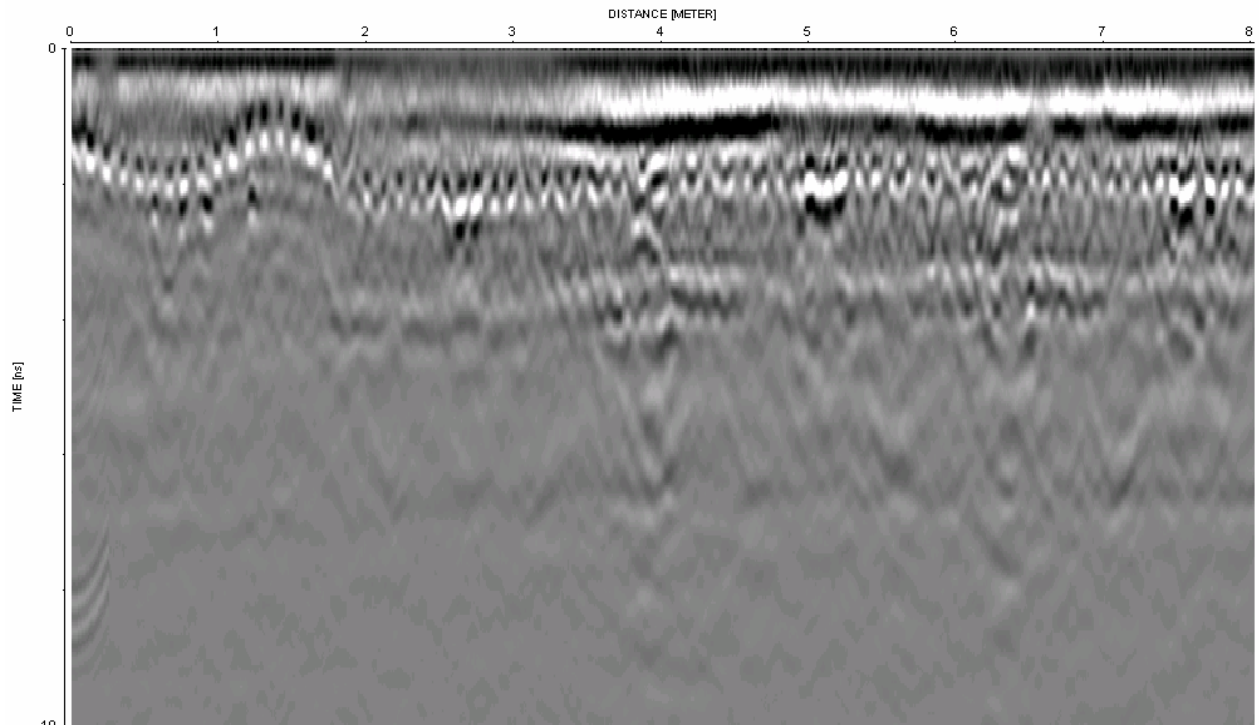
Abbildung 10.1.9: Querprofil, 12.9m ab FÜ Berg, der linke Rand der Darstellung entspricht der Seite Zürich
