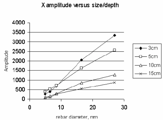
Abbildung 4.1.2: Reflexionsstärke in Abhängigkeit vom Durchmesser und der Tiefe (aus Utsi, 2004)
