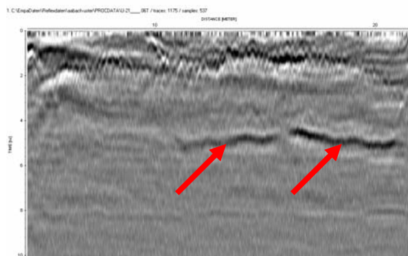
Abbildung 10.5.13: Datensatz der Linie 21
