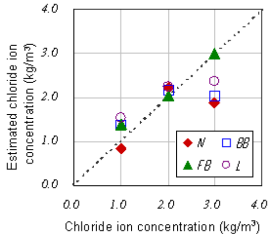
Abbildung 4.2.2: Vergleich von Radarergebnis und Realität für Chloridgehalt für verschiedene Betontypen (aus Arai 2003)
