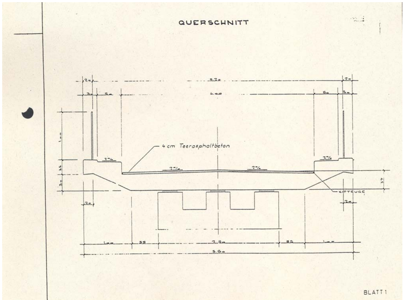
Abbildung 10.4.3: Querschnitt
