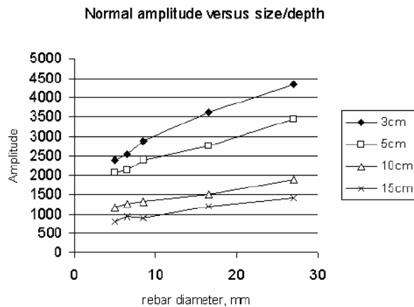
Abbildung.4.1.1: Reflexionsstärke in Abhängigkeit vom Durchmesser und der Tiefe (aus Utsi, 2004)
