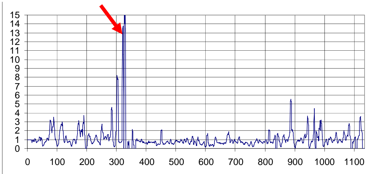
Abbildung 5.6.3: Quotient aus Reflexionsamplituden, Felsenauviadukt
