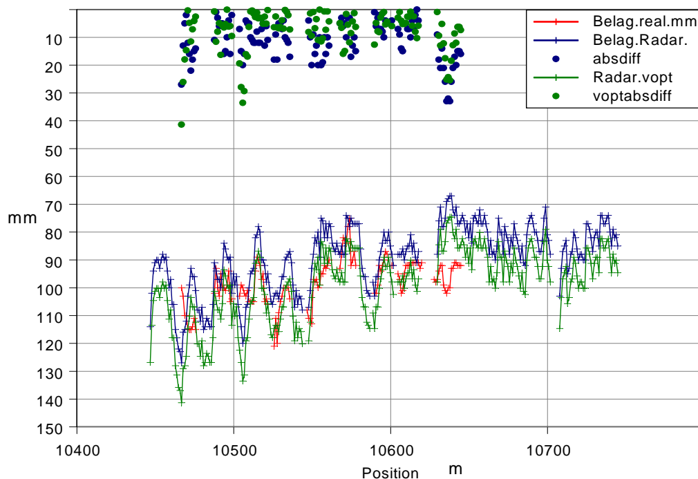
Abbildung 10.3.8: Radarergebnis und Realität für die Asphaltstärke
