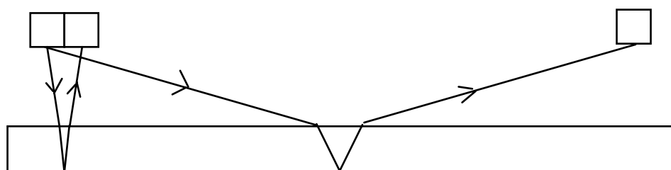
Abbildung 4.3.4: Laufweg des Signals für Hornantennen mit verschiedenen Abständen zwischen Sender und Empfänger
