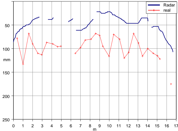
Abbildung 10.5.12: Vergleich Radar – Realität für die Linie B, Eisenüberdeckung oberste Bewehrungslage
