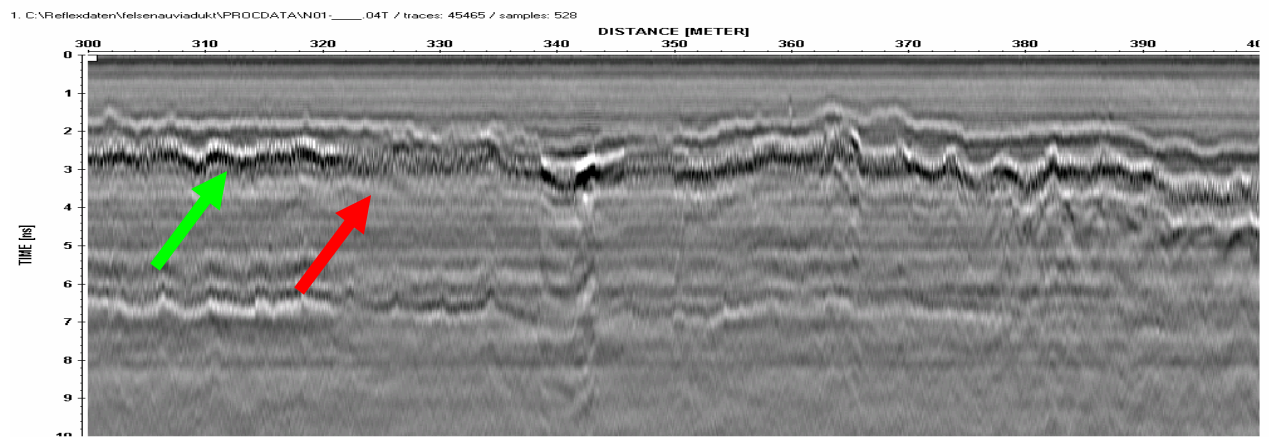
Abbildung 5.6.4: Ausschnitt aus dem Datensatz, Länge 100m, Felsenauviadukt
