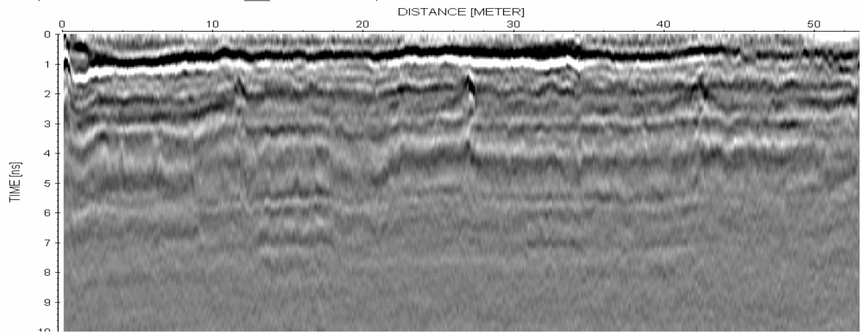
Abbildung 5.3.8: Datensatz von der Überführung Burggasse
