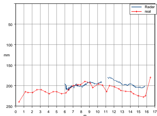
Abbildung 10.5.14: Vergleich Radar – Realität für die Linie A, zweite Bewehrungslage
